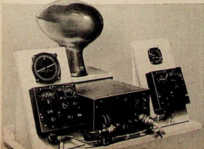
Radlokopaß SCR 269. Auto- matische Pellanlage für Flugzeuge zur Peilung von Rund- funksendern (200 ... 1700 kHz), Funktechnische Werke GmbH.
