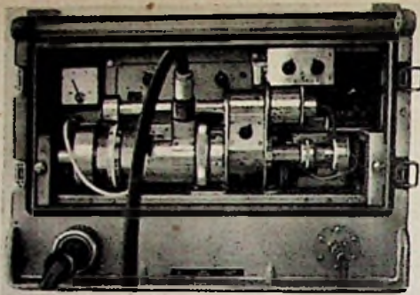
Topkreis-Oszillator 335 ... 420 MHz für eine 6-Kanal-Richtfunk-Anlage der Bundesbahn. Hersteller: Siemens & Halske AG (Vergl. „Richtfunkstrecker bei der Bundesbahn“, S. 262 dieses Heftes)
