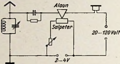
Bild 5. Schaltbild des Kristallverstärkers
