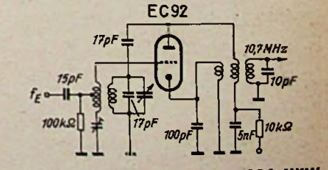
UKW-Oszillator des Braun-Super 220-UKW. Die Röhre EC 92 wird durch eine Katodenrückkopplung für die Zwischenfrequenz entdämpft, damit die Güte des ersten Zf-Bandfilters durch den niedrigen Innenwiderstand der Triode nicht beeinträchtigt wird
