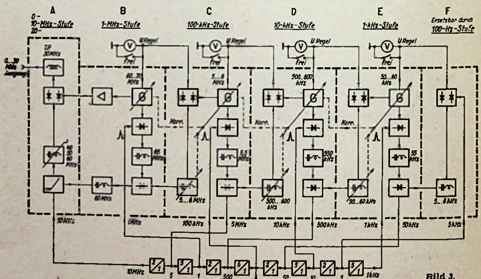
Bild 3. Blockschaltung der Frequenzdekade ND 5
