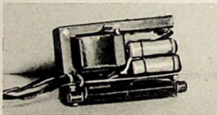
Bild 1. Unterbrecher-(Zehacker-) Aggregat für einen Batterie-Empfänger (Schutzhaube des Aggregates abgenommen). Hersteller des Unterbrechers: Johs. Förderer Söhne, Nidersesbach (Schwarzwald)
