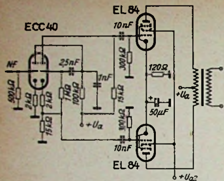
Endstufe beim Siemens-Spitzenuper 54. Zwei Endröhren EL 84 werden im Gegentakt vom zweiten Triodensystem einer Röhre ECC 40 mit Hilfe einer Katodyneschaltung ausgesteuert. Das erste Triodensystem bewirkt eine zusätzliche Nf-Verstärkung wegen der weitgehenden (hier nicht dargestellten) Klangregelung vor dem Gitter dieses Systems
