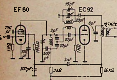
UKW-Eingangsschaltung des Jotha-Mercedes 54. Der UKW-Oszillator liegt hier an einer kapazitiven Brückenschaltung, die den Zwischenkreis von der Oszillatorspannung freihält. Die übliche Zf-Rückkopplung erfolgt über 3nF vom Fußpunkt des ersten Zf-Kreises zum Fußpunkt des Zwischenkreises
