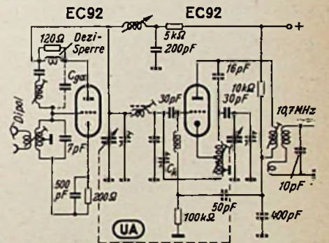
UKW-Doppel-Vorkreissschaltung von Nord-Mende. Der aus der Zusatzspule und C gr gebildete Sperrkreis verhindert das Rückfließen der verstärkten Hochfrequenz zum Gitter. Durch die Kathodenanzapfung des Oszillatorkreises und das richtige Einstellen des Kompensationskondensators C k wird das Gitter der Mischröhre frei von Oszillatortensionen; die Störstrahlung wird dadurch ein Minimum
