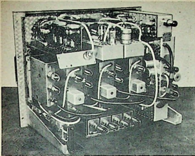
Bild 4. Innenansicht. Infolge der Baukasten-anordnung lassen sich leicht beliebige Frequenzbereiche zusammenstellen
