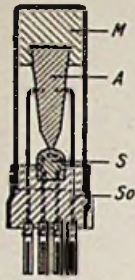
Bild 3. Hörmuschel mit Germaniumdiode und Dipol
