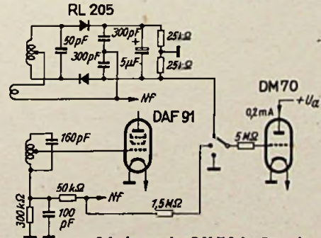
Schaltung der DM 70 im Brandt-Batteriesuper. Das Gitter des Magischen Strichs DM 70 wird mit einer negativen Regelspannung gesteuert. Bei starken Sendern ist daher der Leuchtstrich am niedrigsten (vergl. FUNKSCHAU 1952 Heft 17, Seite 342)
