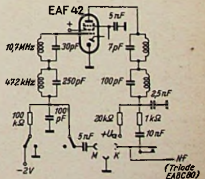
Zusätzliche TA-Verstärkung bei den Saba-Geräten. Magnetische Tonabnehmer werden bei M angeschlossen. Die letzte Zf-Röhre EAF 42 erhält eine negative Vorspannung von -2V und arbeitet dann als zusätzliche Nf-Stufe mit dem 20-kΩ-Anodewiderstand. Kristall-Tonabnehmer werden bei K eingesteckt. Die Schaltbuchse trennt dann die Kopplung zur Anode der EAF 42 auf
