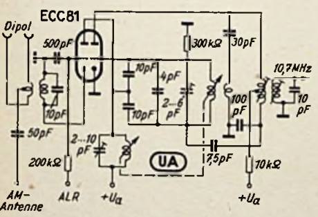
UKW-Eingangsstell der AEG-Super. Je ein System der Röhre ECC 81 dient als geregelte Eingangsstufe in Gitterbassschaltung (Strahlungsfreiheit, keine Neutralisation) und als Oszillatorsystem
