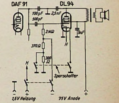
Sparschaltung beim Batterie-Super Braun 100 B. Beim Abschalten einer Heizfadenhälfte der Endröhre wird gleichzeitig der Widerstand zur Erzeugung der Gittervorspannung vergrößert
