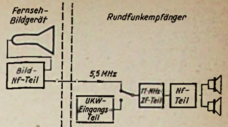
Fernseh-Tonverstärkung beim Krefft Weitfunk W 539. Die Differenzträgerfrequenz von 5,5 MHz aus dem Fernsehbildgerät wird dem auf 11 MHz abgestimmten FM/Zf-Teil des Rundfunkempfängers zugeführt, der die erste Harmonische von 5,5 MHz = 11 MHz ausbleibt und weiterverstärkt
