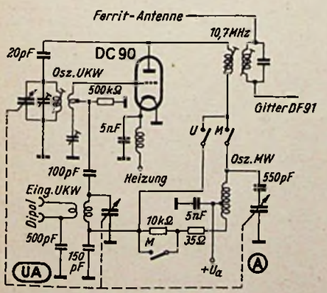
Mischstufe des Akkord-Offenbach U 53. Die Triode dieses Reisesupers DC 90 dient gleichzeitig als UKW-Eingangs- und Oszillatortöhre, und sie wird außerdem zur Erzeugung der MW-Oszillatorfrequenz verwendet
