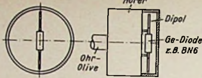
Bild 3. Hörmuschel mit Germaniumdiode und Dipol
