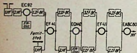
Blockschaltung der Südfunk-Empfänger, Typ Diamant. Die AM-Vorstufenröhre EF 41 dient gleichzeitig als erste Zf-Verstärkerstufe im FM-Kanal. Das Hexodensystem der ECH 41 rückt dadurch an die zweite Stelle im Zf-Verstärker. Dies erlaubt die Unterbringung eines weiteren Zf-Filters, so daß sich für den UKW-Empfang insgesamt 11 Abstimmkreise ergeben
