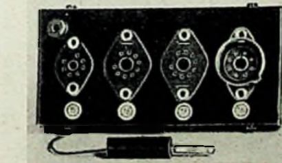
Bild 1. Ansicht des Zusatzgerätes zur Prüfung neuer Röhrentypen
