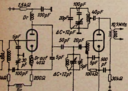
Zwischenbasisschaltung im UKW-Eingangsteil des Kaiser-Super Breslau. Der Eingangskreis ist zwischen Gitter und Katode über einen kapazitiven Spannungsteiler geerdet. Beide Elektroden führen demnach Hf-Spannung. Die Schaltung vereinigt die Vorteile der Gitter- und der Katodenbasisschaltung. Sie ergibt besonders günstige Verstärkung und geringes Rauschen, außerdem wird durch die annähernd erdsymmetrische Anordnung des Eingangskreises die Abstrahlung von Oberwellen der Oszillatorspannung weitgehend vermindert
