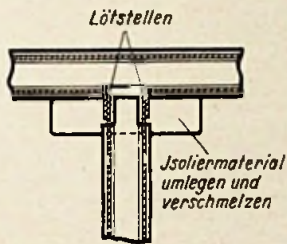
Bild 2. Anschluß der Zuleitung zum Faltdipol
