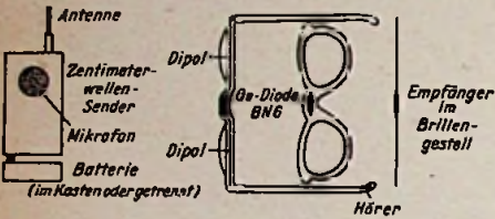
Bild 2. Hörhilfe, bestehend aus einem Zentimeterwellen-Sender und einer Antennenbrille
