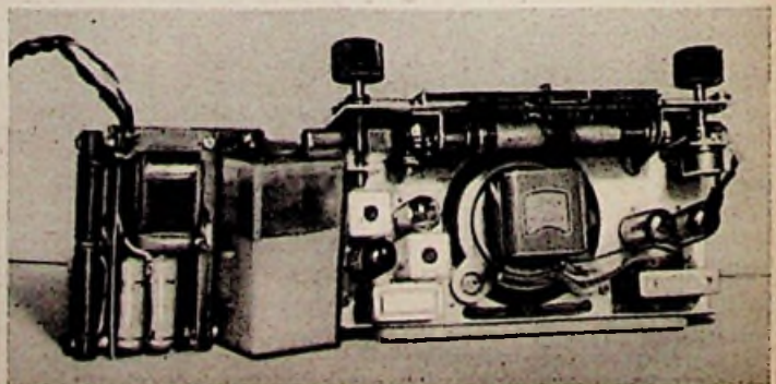
Bild 2. Unterbrecher-Aggregat mit Klein-Akkumulator und Empfängerchassis (ohne Koffer)
