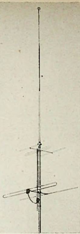
Bild 2. Kombinierte Antenne für den Empfang der Bereiche UKW, Kurz-, Mittel-, Lang- und Fernsehen (Siemens)
