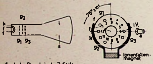
Sockel: Duodekal, 7 Stifte (I. V. — innere Verbindung)
