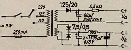
Netzteil für einen Brandt-Batteriesuper. Durch getrennte Gleichrichter und Siebketten für Heiz- und Anodenspannungen wird die Stromversorgung des Empfängers für beide Betriebsarten (Netz und Batterie) besonders einfach
