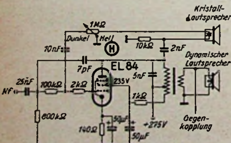
Endstufe mit der Röhre EL 84 im Telefunken-Super Concertino. Der Kristall-Hochtonlautsprecher ist über einen Hochpaß, bestehend aus 2 nF und 10 kΩ, angekoppelt. In Stellung „hell“ des Höhenreglers ist der Lautsprecher voll wirksam, beim Übergang aus Stellung „dunkel“ wird er allmählich abgeschaltet und stattdessen tritt eine tonblende Wirkung durch den 10-nF-Kondensator am Steuergitter der EL 84 ein.— Beim Ausgangsübertrager wird eine Brummkompensationsschaltung angewendet. Am Schirmgitter der Endröhre werden auch die Anoden- und Schirmgitterströme sämtlicher Vorröhren abgenommen
